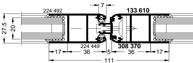
ASS 28 SC.NI
