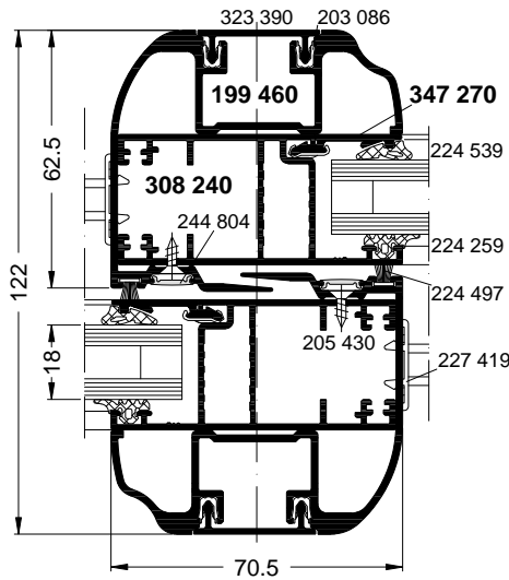
ASS 32.NI
