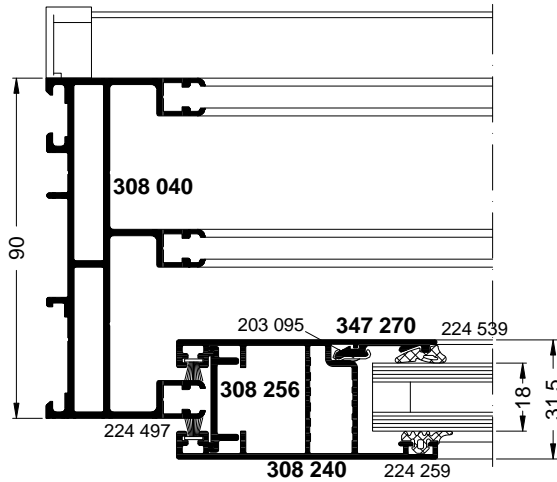
ASS 32.NI
