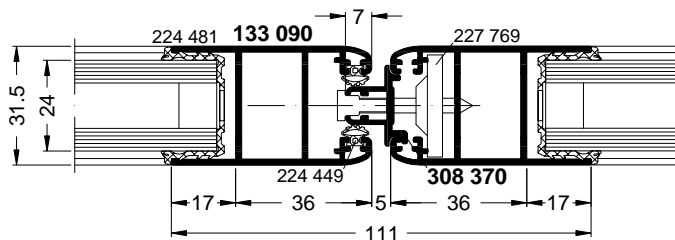
ASS 32 SC.NI
