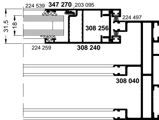
ASS 32.NI
