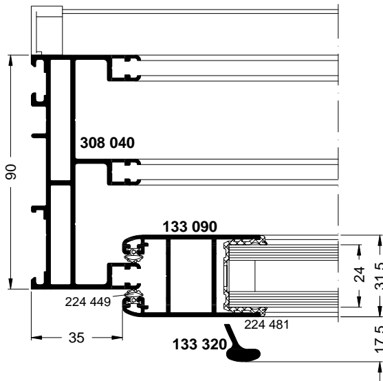
ASS 32 SC.NI
