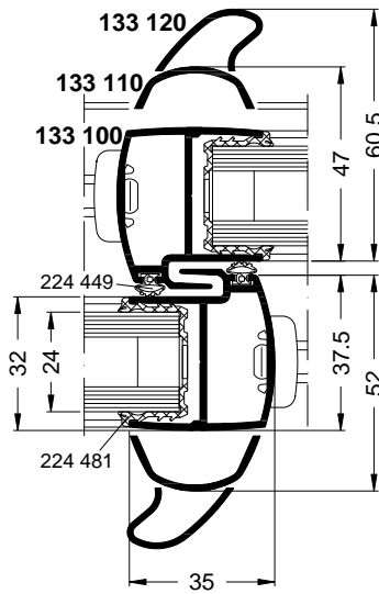
ASS 32 SC.NI
