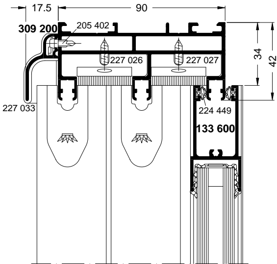
ASS 28 SC.NI
