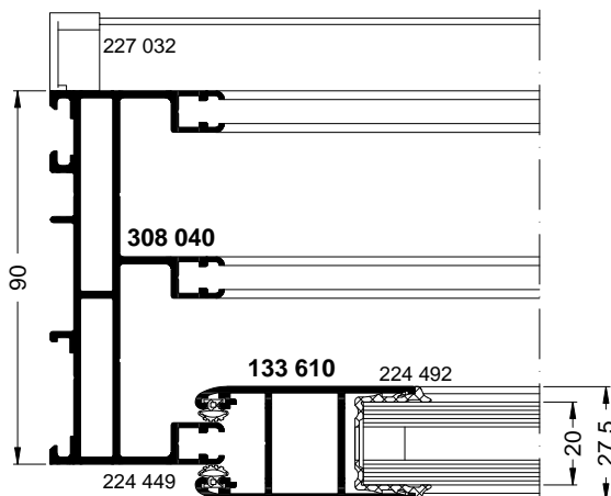
ASS 28 SC.NI
