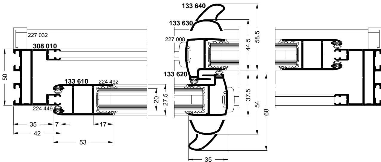
ASS 28 SC.NI
