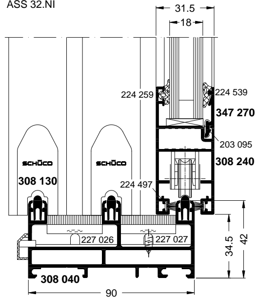
ASS 32 SC.NI
