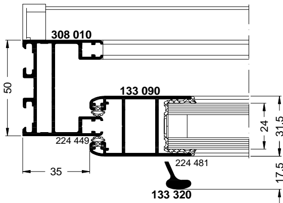
ASS 32 SC.NI
