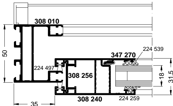
ASS 32.NI
